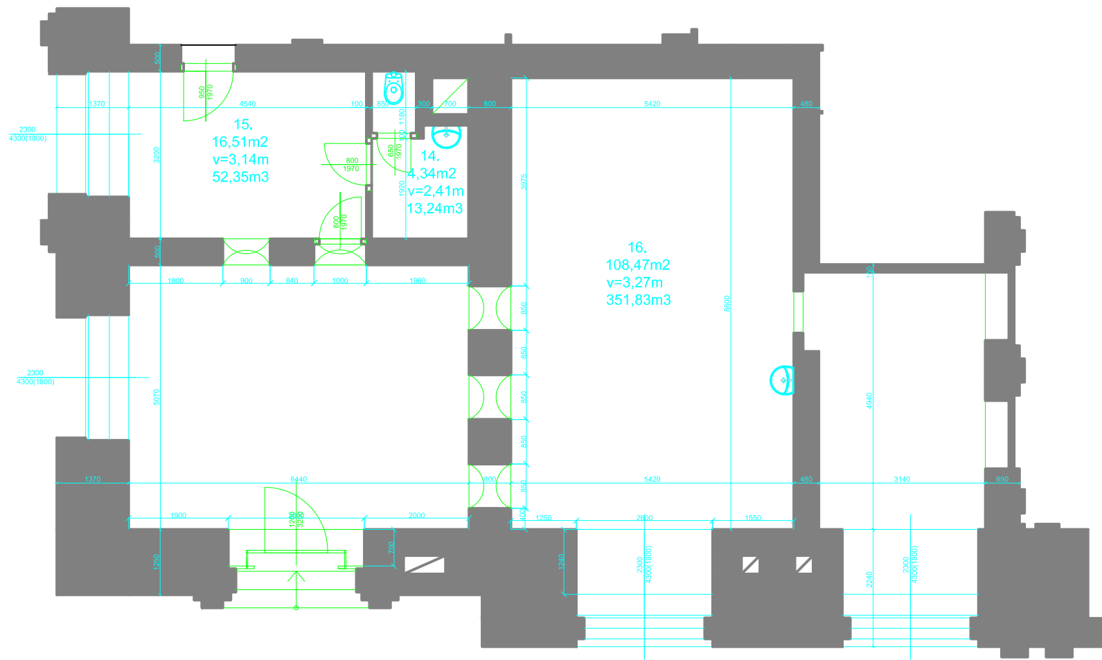
Národní dům na Vinohradech Praha 2, nám. Míru 9 Přízemí- obchodní prostory M-1:100
